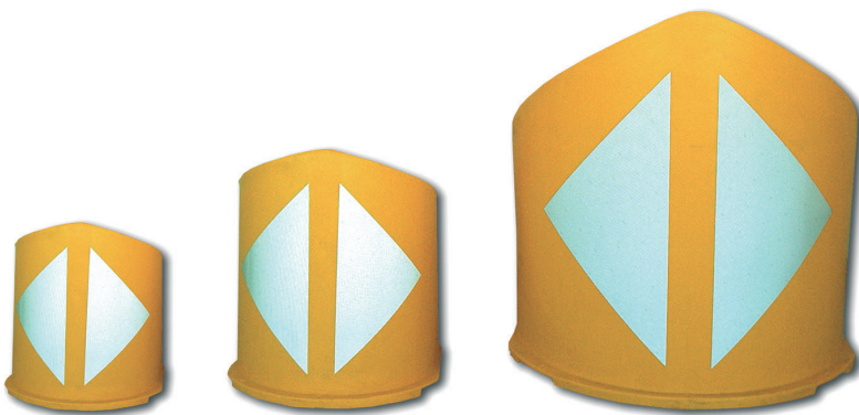
A471 Ø 1000 x h 1220 B471 Ø 1500 x h 1340 C471 Ø 2000 x h 1475 Deviatore di corsia in polietilene. Con Frecche Rifrangenti in Classe 2 Colore: giallo stradale
