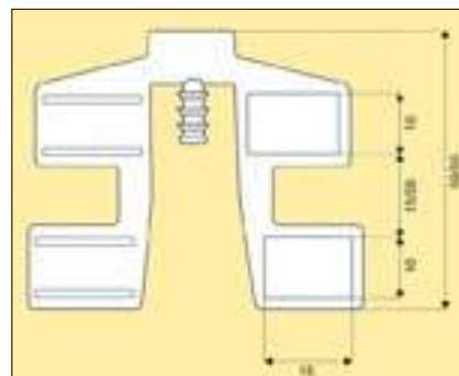
Delineatore per New Jersey con 4 catadiottri 10x15 cm 457 Senza spinotto per installazione 457S Con spinotto per installazione
