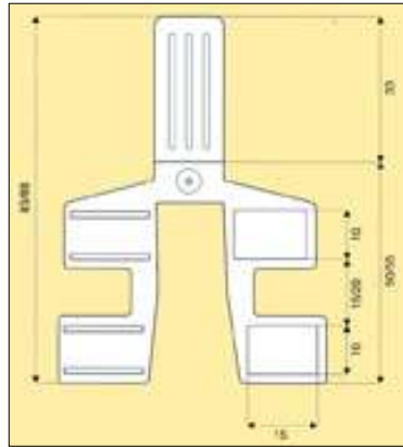
837 Staffa per delineatore per New Jersey
